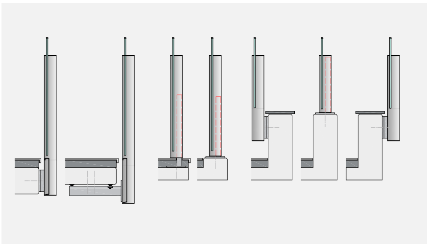
Montageanbindung
