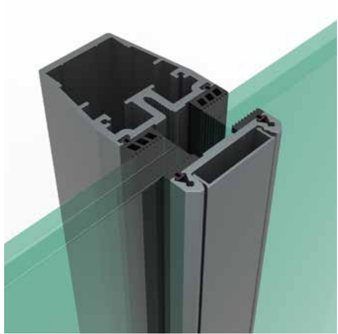
Designgeprägte Glaslagerung ohne optisch störende Glasklemmhalter
